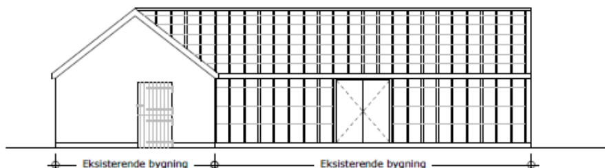
Facade af orangeri mod vest mål 1:100
