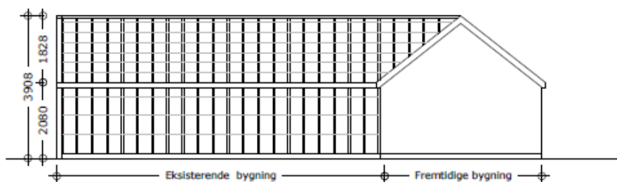
Facade af orangeri mod syd
